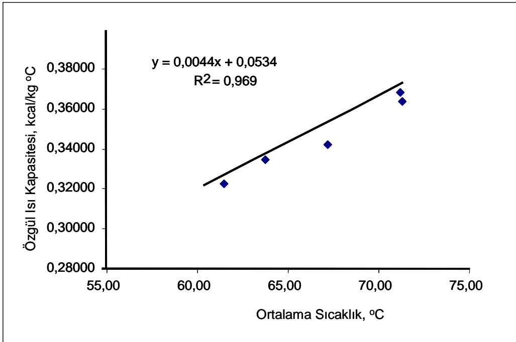
Şekil. Panetti Özgül Isı Kapasite Karakteristiği.
