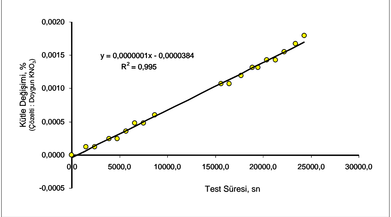
Şekil. Panetti Su Buharı Difüzyonu – Test Örneği Kütle Değişimi Karakteristiği
